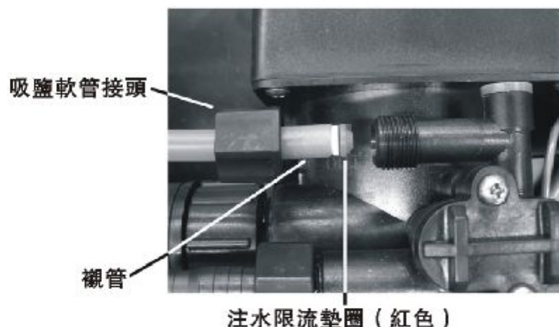
（圖三） 正確的安裝方法
